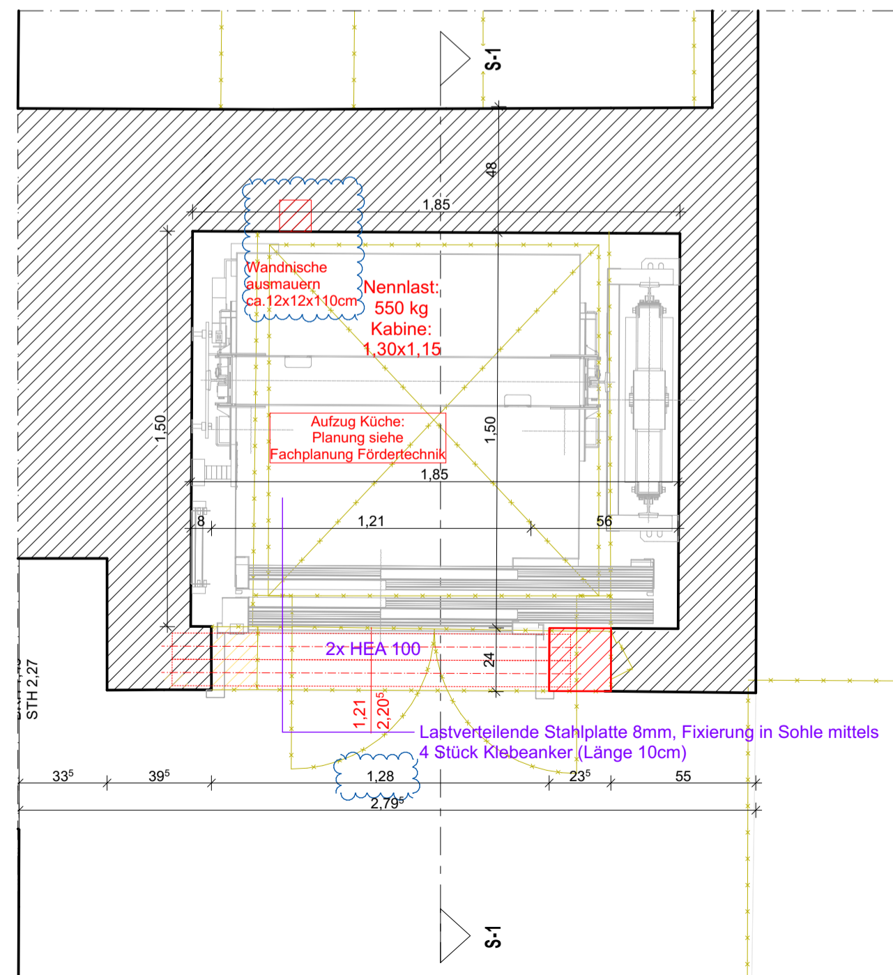
Grundriss KG
