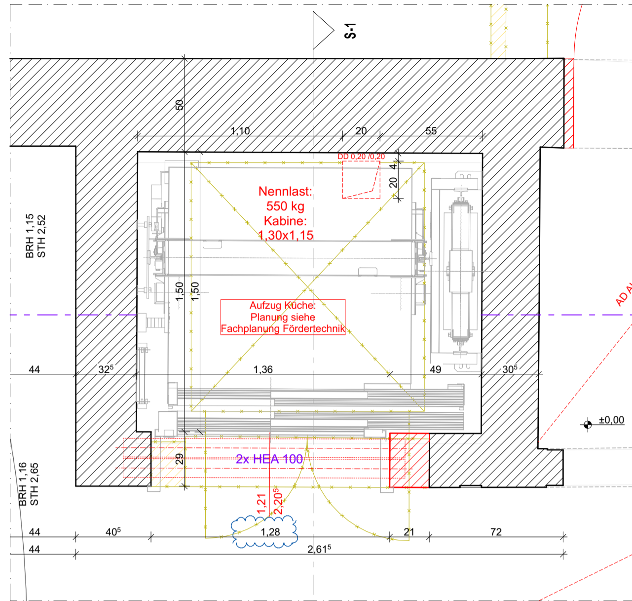
Grundriss EG
