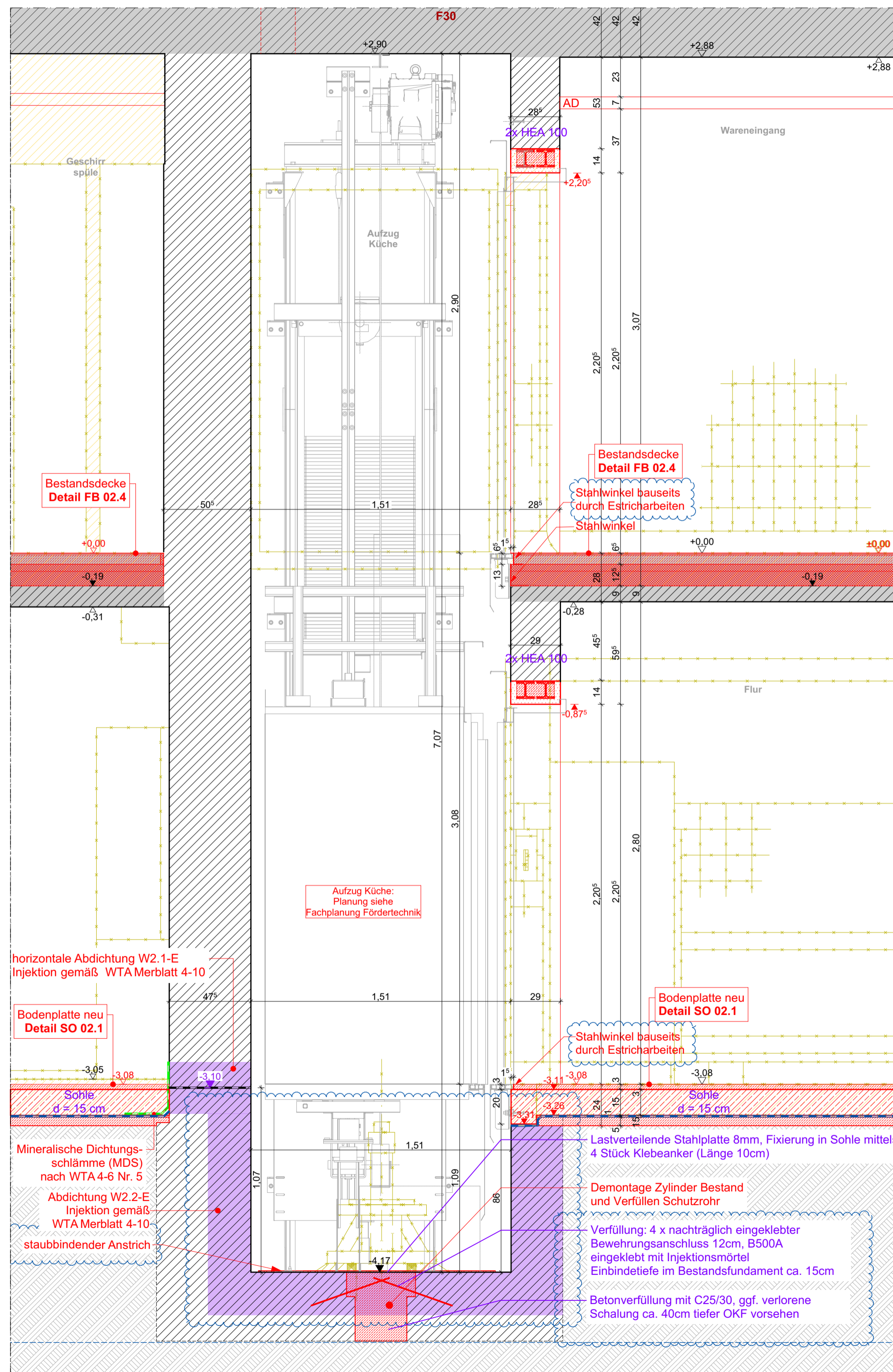
Schnitt
